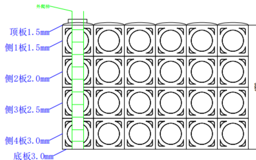
水箱正视图6000×4500×4000mm
