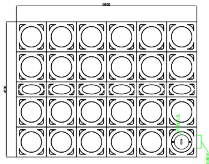
水箱俯视图6000×4500×4000mm
